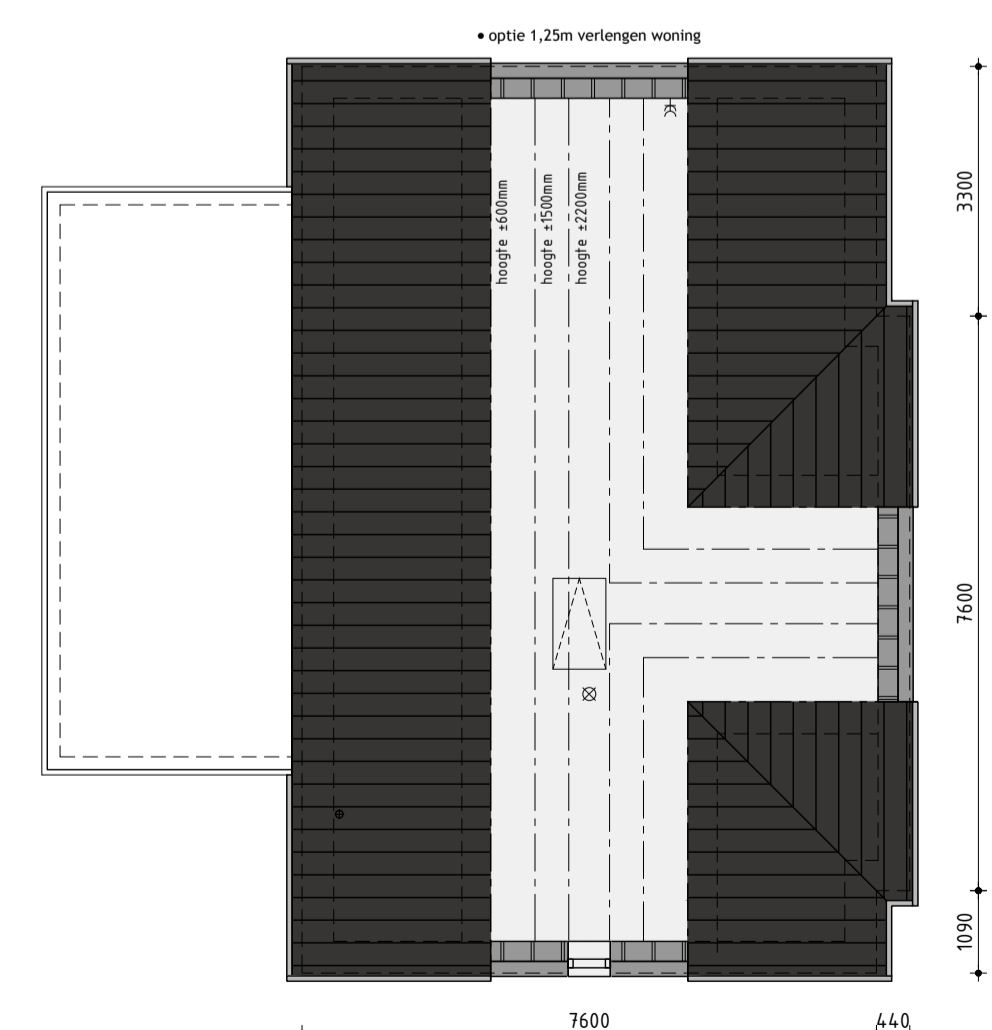
2de Verdieping
