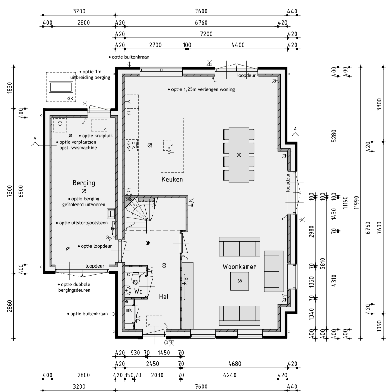
Begane grond
