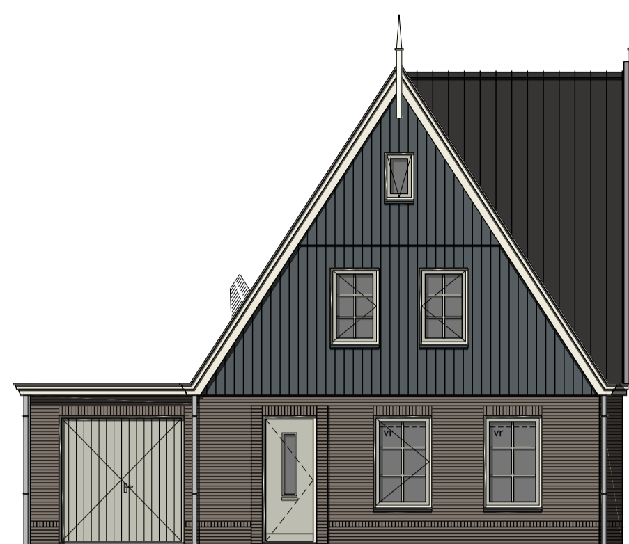
Voorgevel
