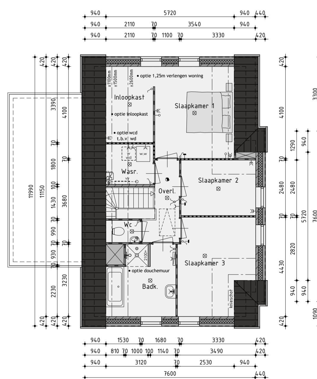
1ste Verdieping
