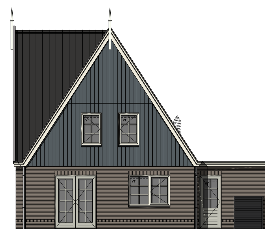
Achtergevel
